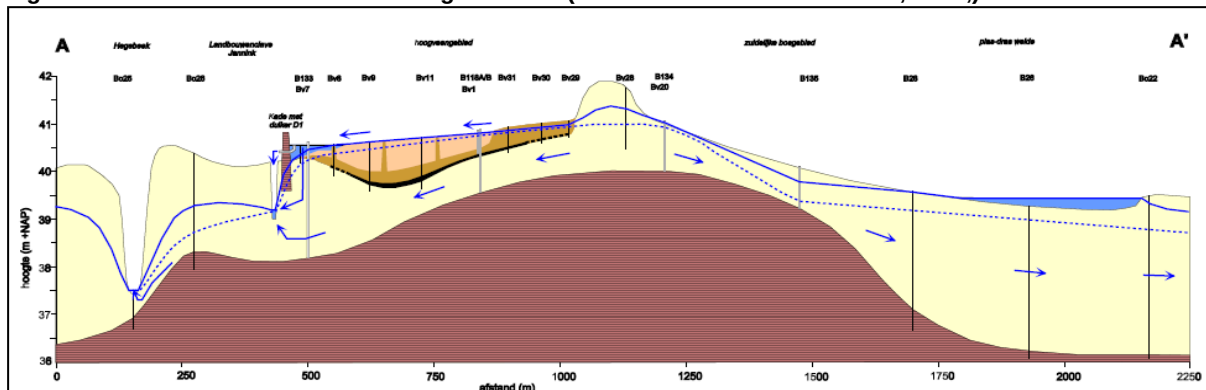
Figuur 3.1. Doorsnede noord-zuid hoogveenkern (Bron: Bell & van 't Hullenaar, 2004,).
